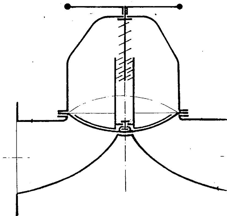
DIFRAGMA (MEMBRÁN) SZELEP
