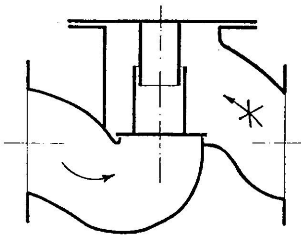
VISSZACSAPO SZELEP
