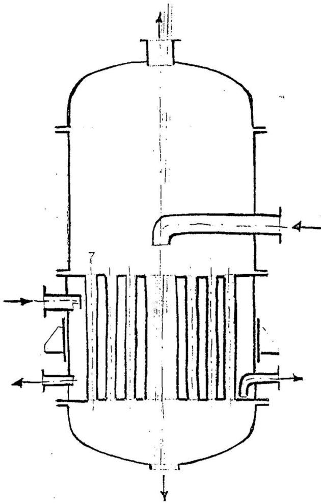
Robert bepárló
