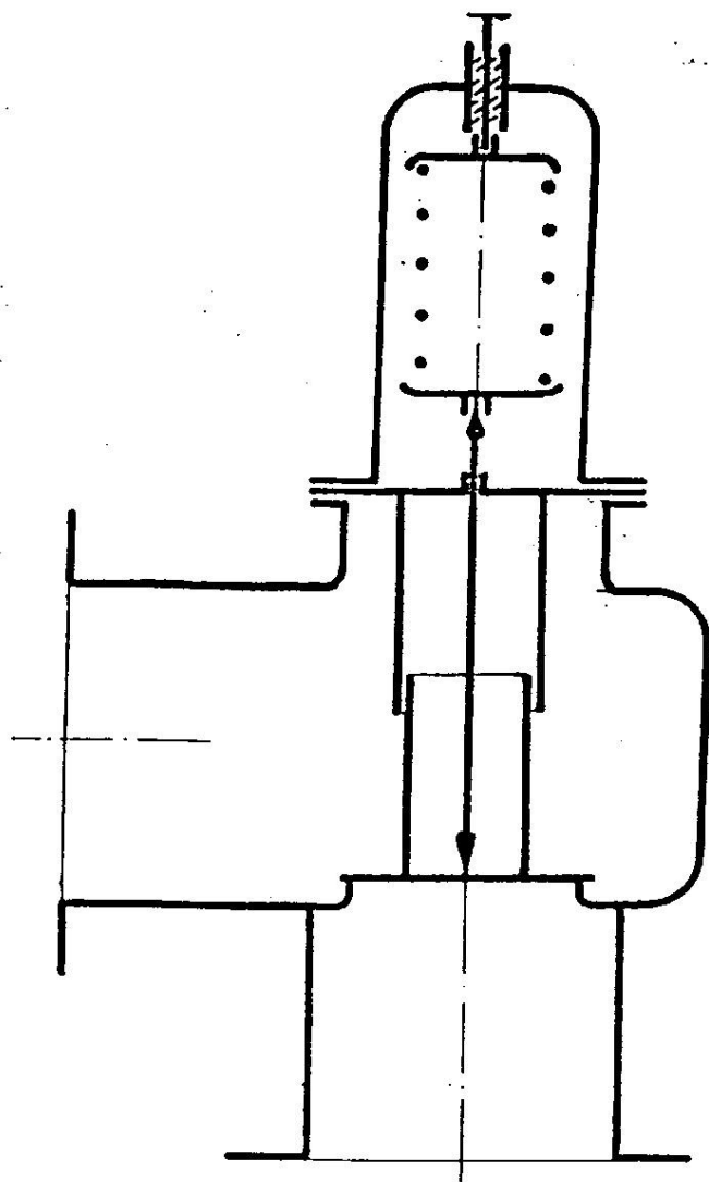
RUGÓTERHELÉSŰ BIZTONSÁGI SZELEP
