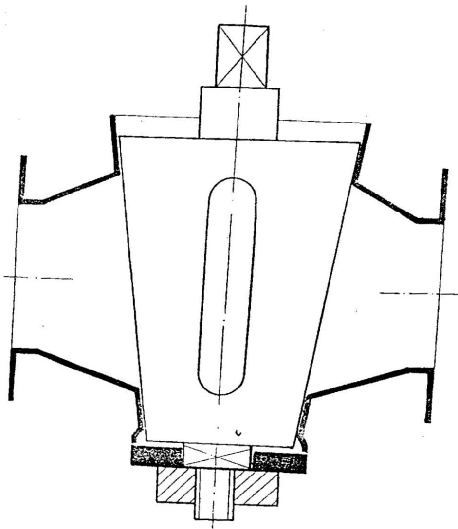
TÖMSZELENCE NÉLKÜLI CSAP
