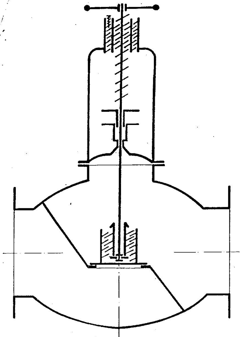
KÜLSŐ MENETES SZELEP
