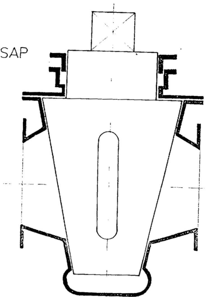
TÖMSZELENCÉS CSAP
