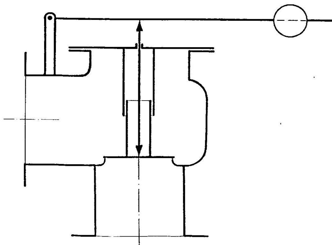
SÜLYTERHELÉSŰ BIZTONSÁGI SZELEP
