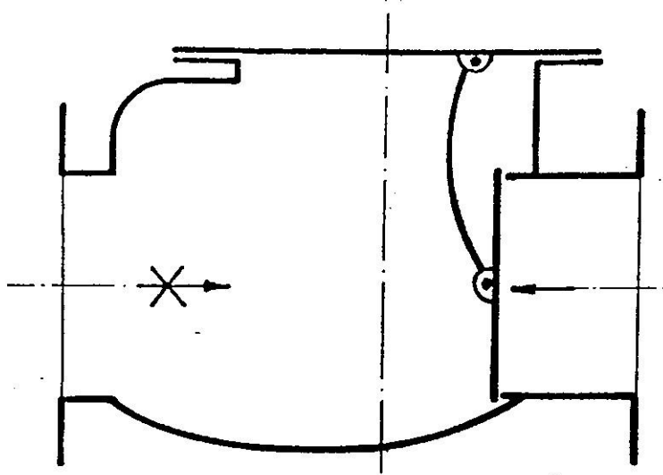
TORLÓCSAPPANTYÚ
